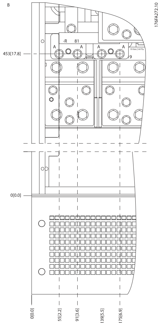
Disegno 3.13: Posizione dei collegamenti dell'alimentazione in custodie IP21 (NEMA tipo 1) e IP54 (NEMA tipo 12) (dettaglio B)
