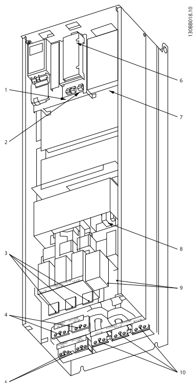
Disegno 3.39: Custodia compatta IP 00 (telaio) con sezionatore, fusibile e filtro RFI, telaio di taglia D4
