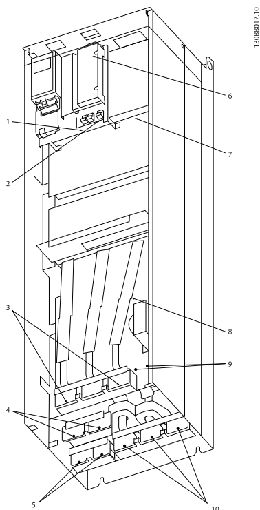
Disegno 3.38: Custodia compatta IP 00 (telaio), telaio di taglia D3
