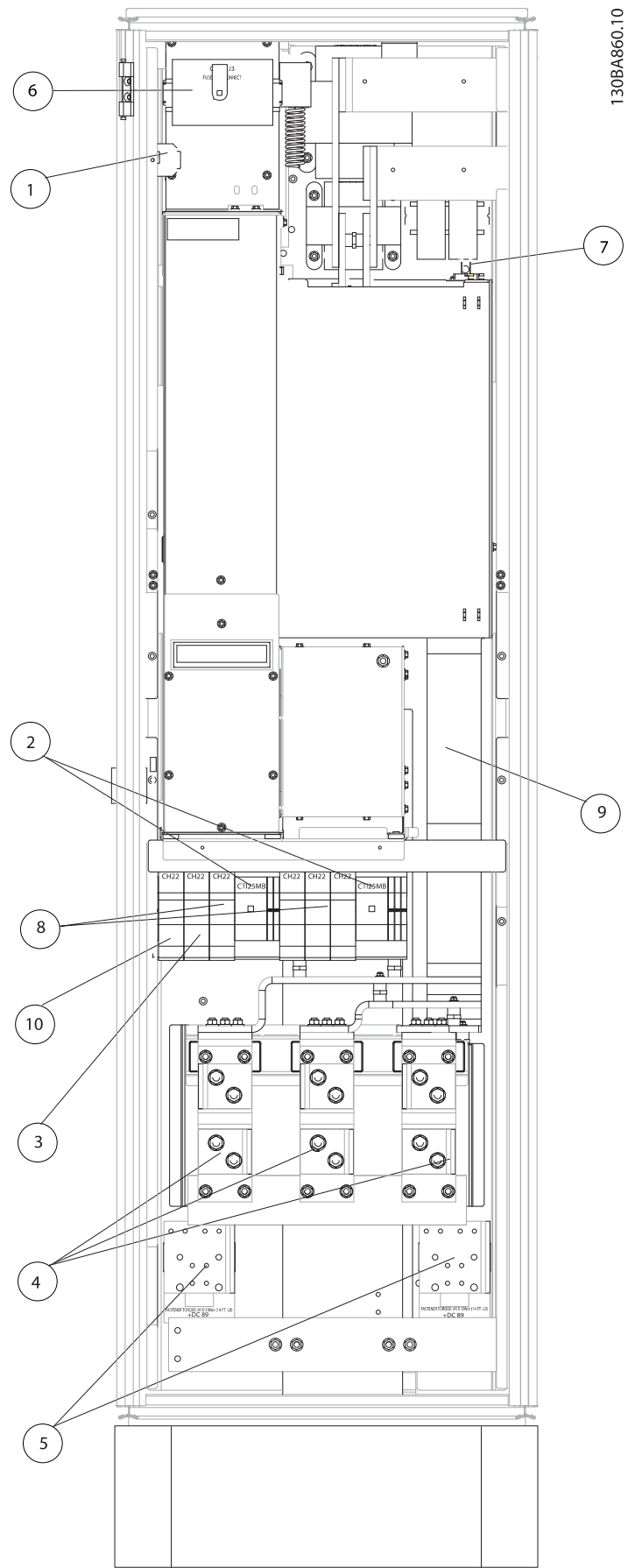
Disegno 3.45: Armadio rettificatore, telaio di taglia F1, F2, F3 e F4
