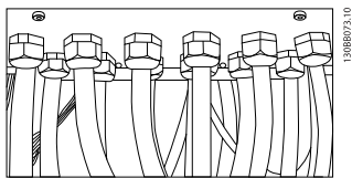
Disegno 3.25: Esempio di corretta installazione della piastra passacavi.
