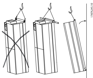
Disegno 3.24: Metodo di sollevamento per montare il convertitore di frequenza a parete
