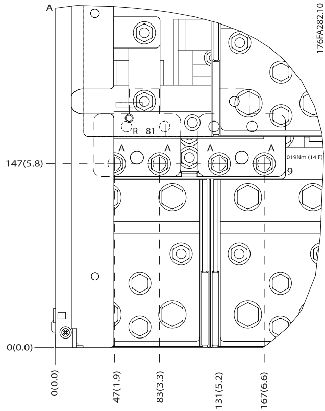
Disegno 3.16: Posizioni dei collegamenti dell'alimentazione in custodie IP00
