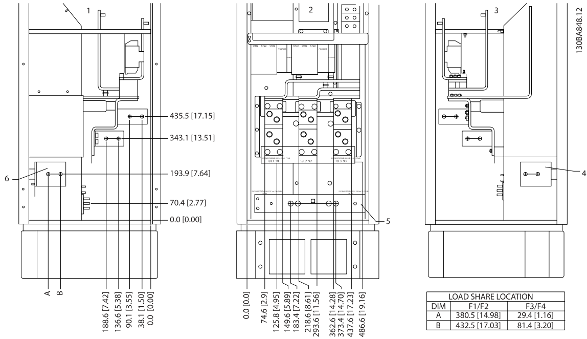
Disegno 3.21: Posizione dei morsetti - raddrizzatore (vista dal lato sinistro, frontale e dal lato destro)
