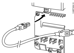
Disegno 4.10: Per collegamenti con cavo di controllo, vedere la sezione Morsetti di controllo .
