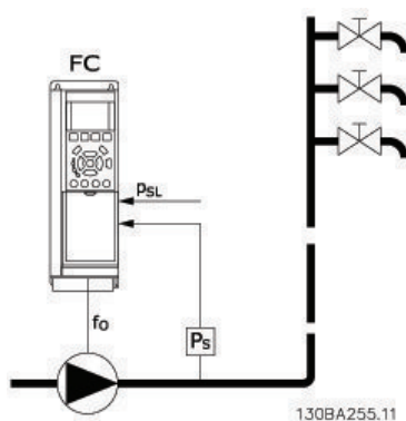
Disegno 3.57 Legenda: FC=convertitore di frequenza; fo=frequenza in uscita; Ps=P sistema; Psl=P setpoint
