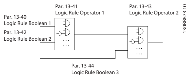
Disegno 3.38 Regole logiche
