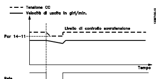
Disegno 3.41 Backup dell'energia cinetica, guasto di rete breve.
