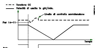
Disegno 3.39 Rampa di decelerazione controllata - guasto di rete breve. Rampa di discesa fino all'arresto seguita da una rampa di salita fino al riferimento.
