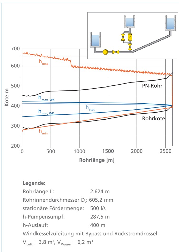
Abb. 5: Druckhöhenlinie von dynamischen Druckänderungen nach Pumpenausfall
