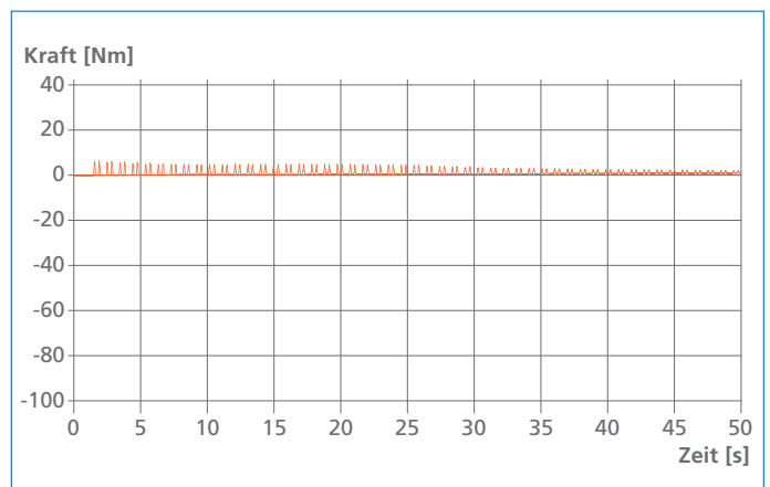
Abb. 27: Längskraft auf L8 im geschützten System „Regenwetterleitung“
