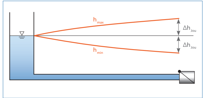
Abb. 10: Einhüllende der Druckhöhen für Schließzeiten größer als die Reflexionszeit T_r
