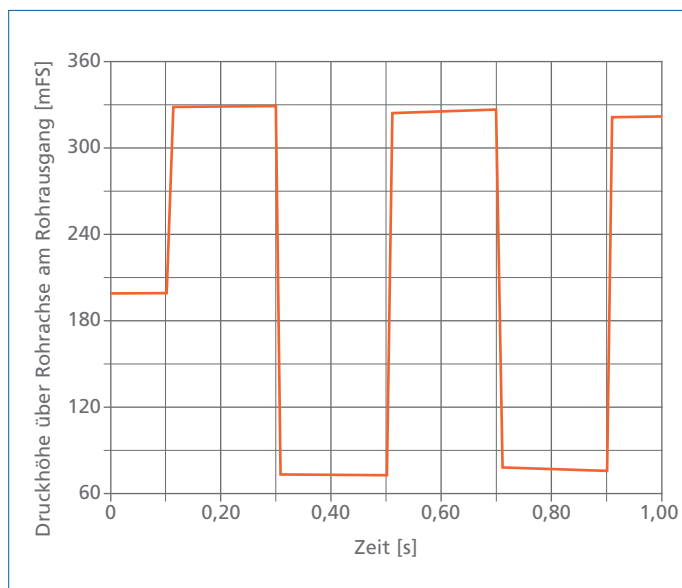
Abb. 9: Druckhöhe vor dem Schieber. Gegenüber der in Abb. 8 dargestellten Situation sind ganz kleine Abweichungen erkennbar. Die Druckflanken sind z. B. wegen der endlichen Schließzeit von D_s = 0,01 s nicht ganz senkrecht. Die Druckplateaus sind als Folge der Reibung nicht vollständig waagerecht – auf diese Erscheinung wird im Kapitel „Der Geltungsbereich der Joukowsky-Formel“ auf Seite 12 noch näher eingegangen.
