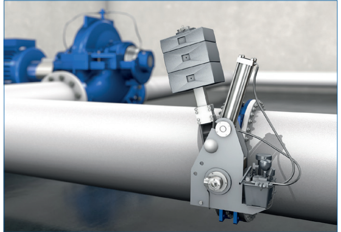
Abb. 20: KSB Rückschlagklappe Dualis mit hydraulischer Antriebseinheit
