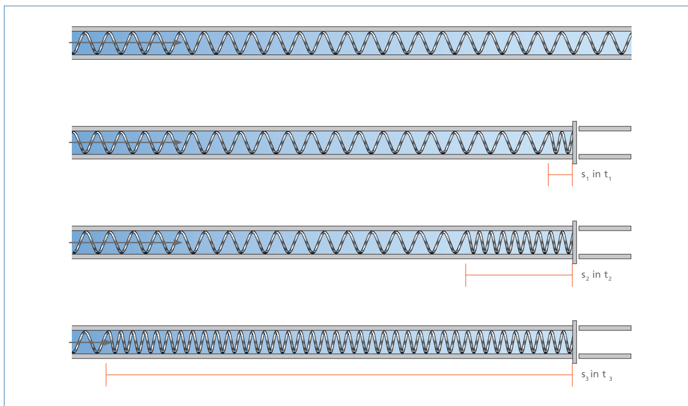
Abb. 7: Plötzliches Schieberschließen, veranschaulicht durch eine schwere Stahlfeder
