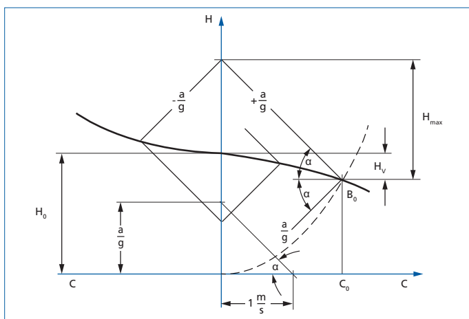
Abb. 12: Grafisches Verfahren nach Schnyder-Bergeron
