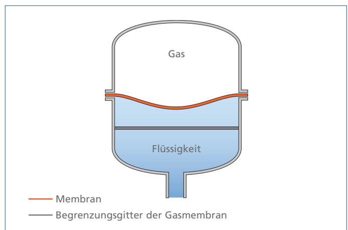
Abb. 14: Schema eines Membranwindkessels
