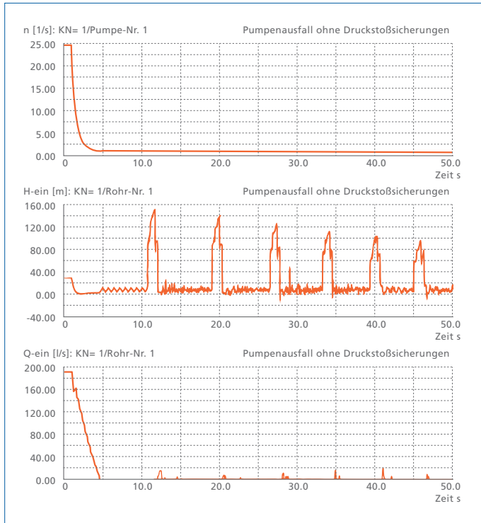
Abb. 24: Zeitverläufe des ungeschützten Systems „Regenwetterleitung“
