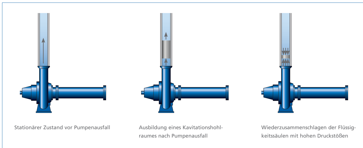
Abb. 6: Makrokavitation nach Pumpenausfall
