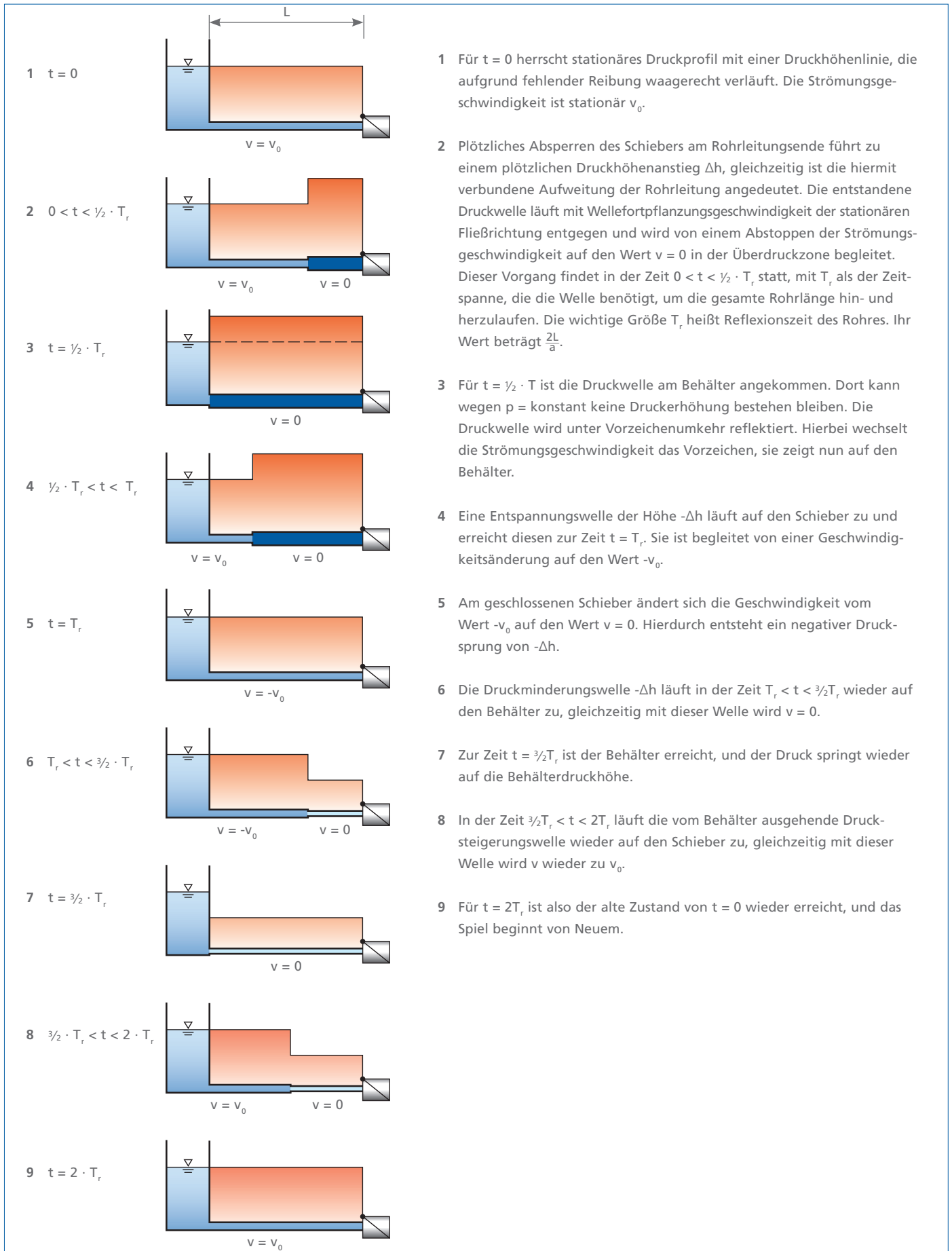
Abb. 8: Druck- und Geschwindigkeitswellenverlauf in einer einsträngigen, reibungsfreien Rohrleitung nach plötzlichem Absperren. Die Zonen mit stationärer Druckhöhe sind mittel, mit Druckerhöhung dunkel, mit Druckabsenkung hell schattiert. Die Aufweitung und Einschnürung der Rohrleitung infolge Druckerhöhung beziehungsweise Druckabsenkung ist angedeutet. Zur Größenordnung: Das Volumen von Wasser verringert sich bei einer Druckerhöhung um 100 bar um etwa 0,5 %.
