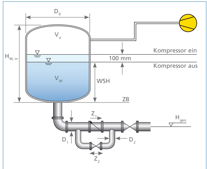
Abb. 13: Schema eines Kompressorkessels Zur Vermeidung von zu hohen Drücken beim Rückschwingen des Kesselwassers ist gegebenenfalls eine Rückschlagklappe mit gestrohltem Bypass in der Anschlussleitung erforderlich.
