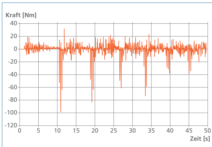
Abb. 25: Längskraft auf L8 im ungeschützten System (ohne Druckstoßsicherungen) „Regenwetterleitung“
