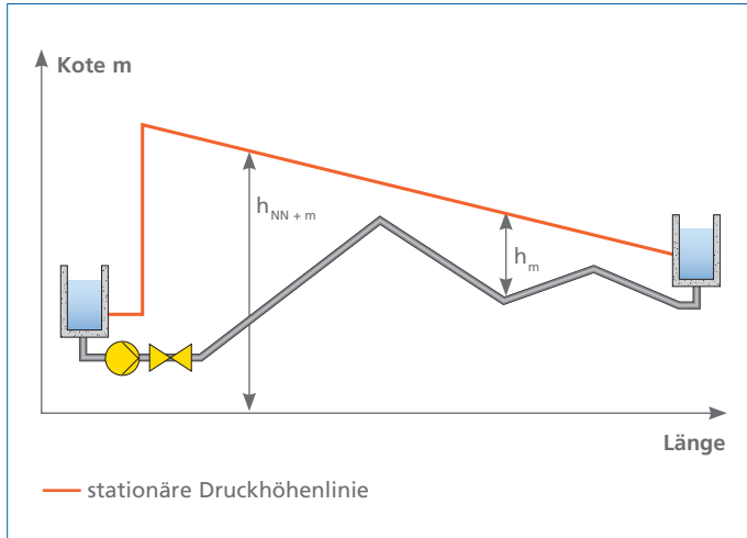
Abb. 4: Zur stationären Druckhöhenlinie einer Pumpanlage
