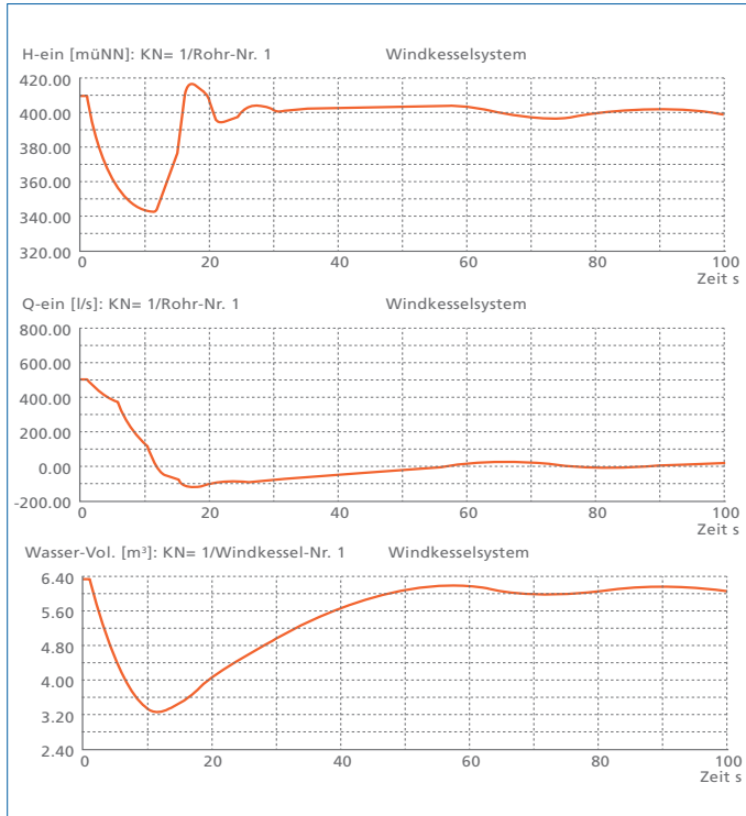
Abb. 21: Zeitverläufe des Beispiels „Fernwasserleitung“ (Abb. 5), gezeigt werden die zeitabhängigen Druckhöhen- und Volumenstromverläufe des mit Windkesselanlage geschützten Systems (Druckhöhen in müNN)
