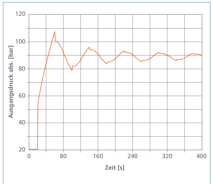
Abb. 11: Druckverlauf am Ausgang einer 20 km langen Rohrleitung nach plötzlichem Schieberschließen. Berechnungsparameter: DN 300, k = 0,02 mm, Eingangsdruck 88 bar konstant, Q = 250 l/s, Fördermedium Rohöl mit \rho = 900 \text{kg/m}^3
