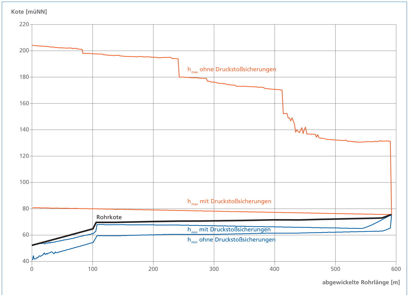
Abb. 28: Druckeinhüllende des geschützten und ungeschützten Systems „Regenwetterleitung“
