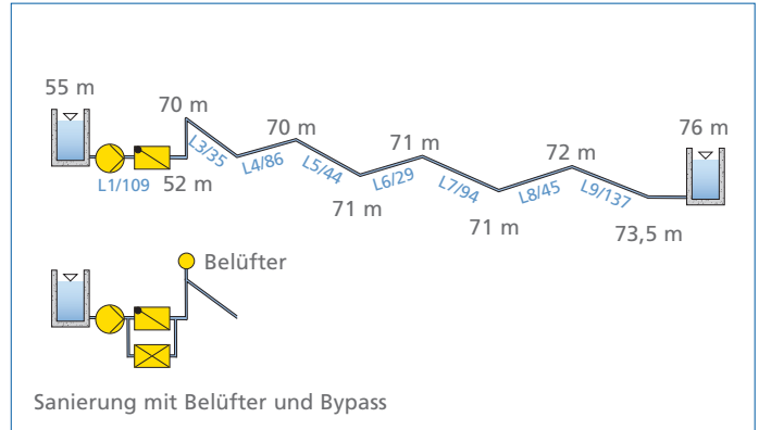
Abb. 22: Schema des Beispiels „Regenwetterleitung“
