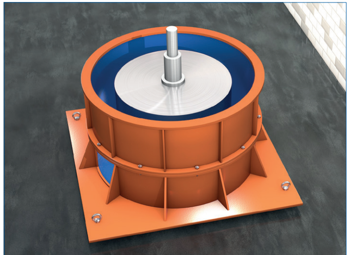
Abb. 17: Vertikal angeordnete Schwungscheibe (Antrieb über Gelenkwelle, D = 790 \text{ mm} )
