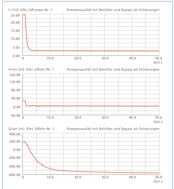
Abb. 26: Zeitverläufe des geschützten Systems „Regenwetterleitung“
