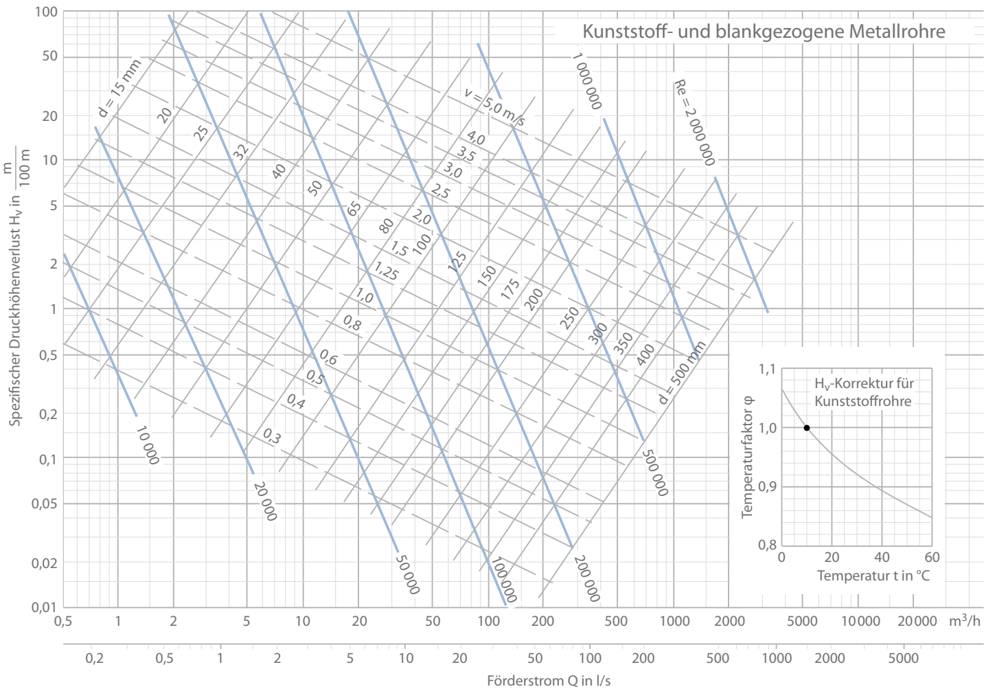
Abb. 5 Druckh henverlust: Druckh henverluste H_v f r hydraulisch glatte Rohre ( K = 0 ) (f r Kunststoffrohre bei t \neq 10^\circ\text{C} mit Temperaturfaktor \phi zu multiplizieren)
