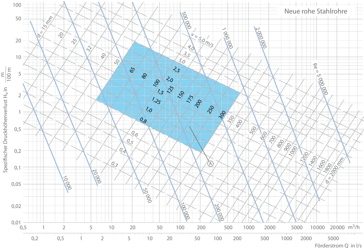
Abb. 3 Druckhöhenverlust: Druckhöhenverluste H_v für neue Stahlrohre ( k = 0,05 mm ) siehe auch Feld (A) im Anhang unter Druckhöhenverlust Abb. 1
